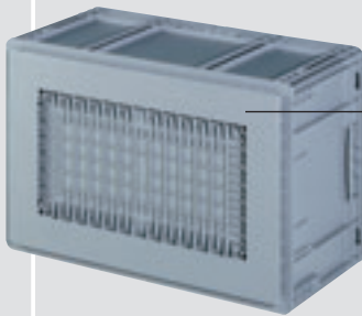
Standard-Boden für störungsfreie und sichere Einlagerung im AKL (max. Inhaltslast 35 kg)
