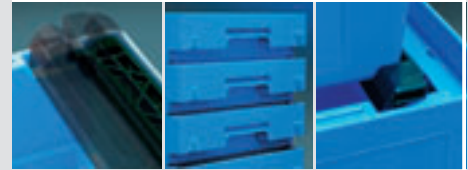
Stapelbügel für leeres oder befülltes Stapeln durch Drehung um 180° und Arretierung
