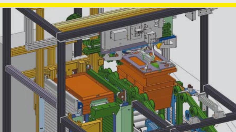
▲ ▼ Detail einer Deckelmaschine
