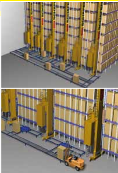
Magazynowanie palet
